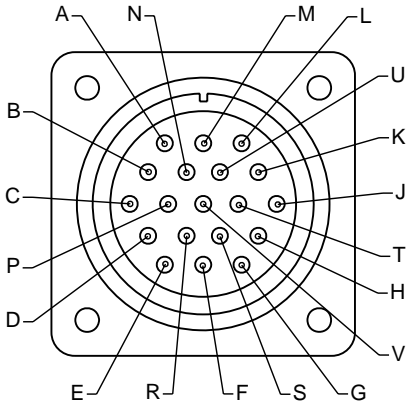
VB4-T Tool Side (MS3102E22-14S)
