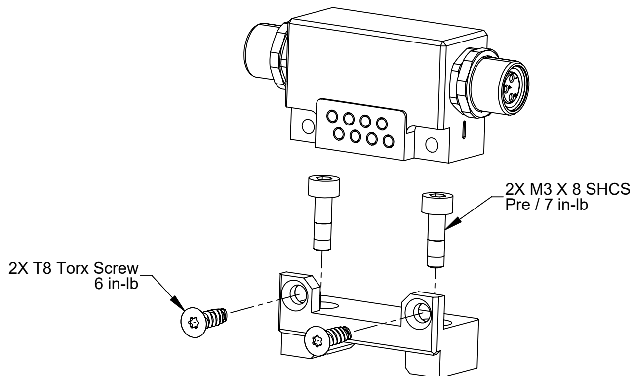
9120-ML6-T Tool Module
